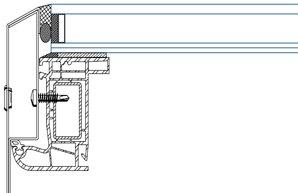
Die BEWILUX-Glasarchitektur-FLATLIGHT Konstruktion
