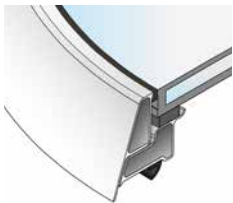
Wärmedämmverglasung 2-fach U-Wert 1,1 W/m 2 K
